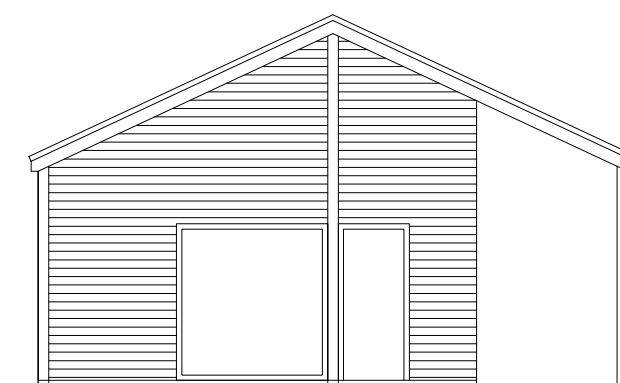
SEVERNÍ POHLED
